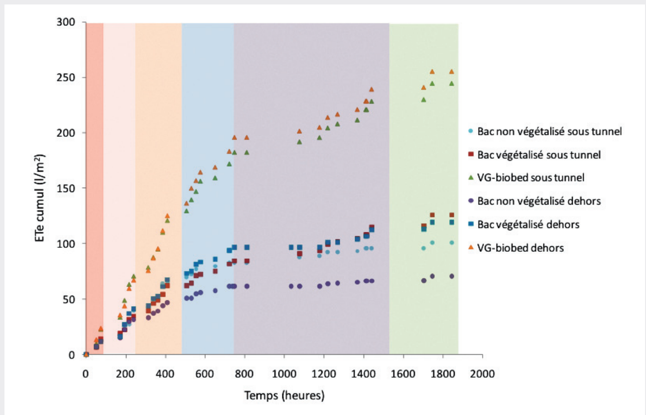
Fig. 3 Évapotranspiration efficace cumulée (ETe cumul) d'un biobac, d'un phytobac et du VG-biobed en fonction des arrosages et de leurs emprises au sol Effektive kumulierte Evapotranspiration (ETe cumul) von Biocontainer ohne (Biobac) und mit Bepflanzung (Phytobac) sowie VG-Biobed™ [8]
